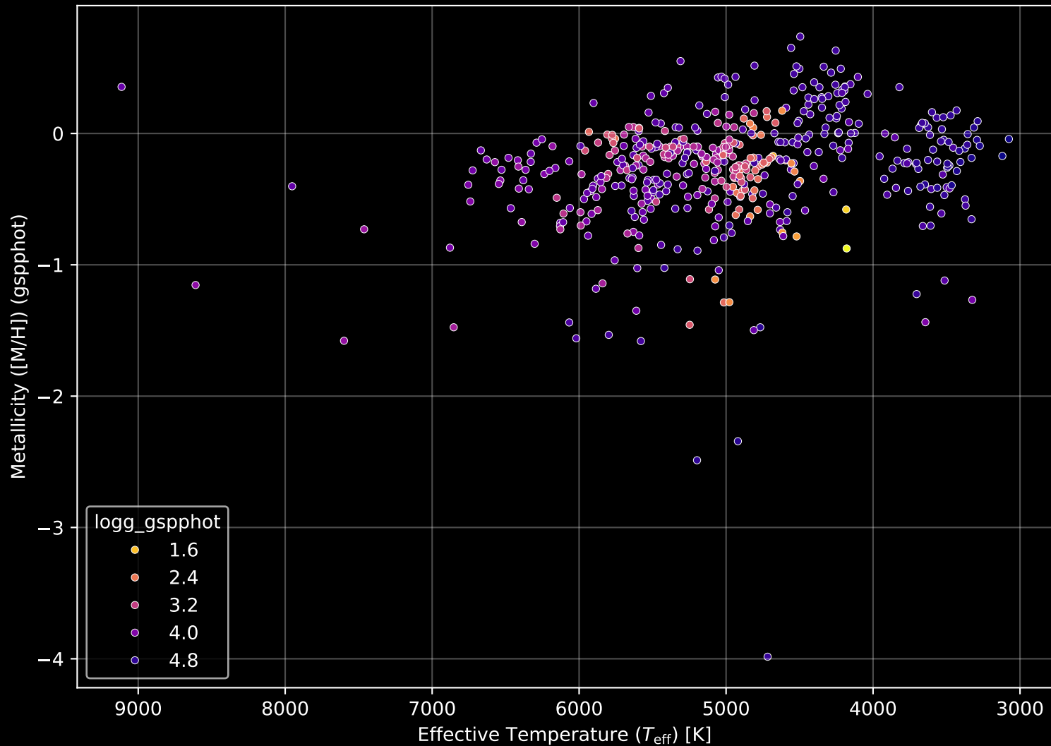
APOGEE DR17 Field: [080+45] Stellar Population Parameters (n= 518)
